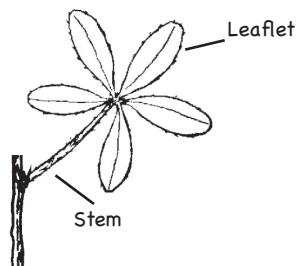
Palmate
