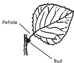
Simple
